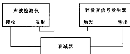
图 3 幅值测量级线性的检定装置示意图
