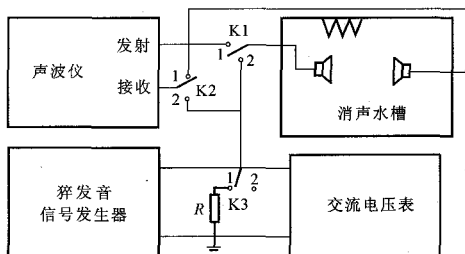
图5 声波检测仪测量范围的检定装置示意图
